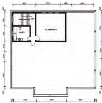
Tercer Planta
