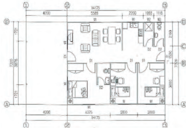
Plano
