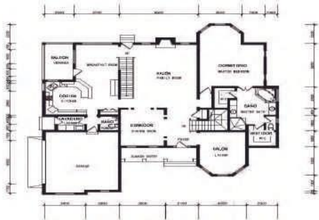
Plano Primera Planta
