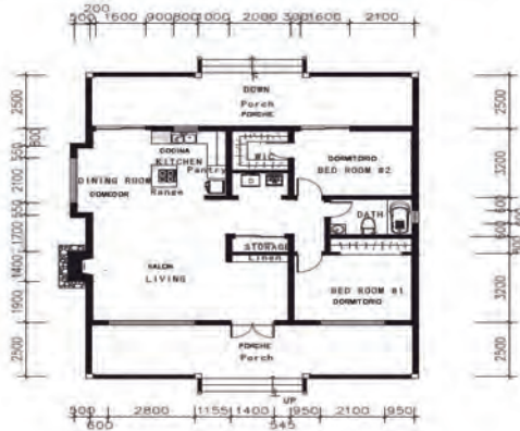
Plano
