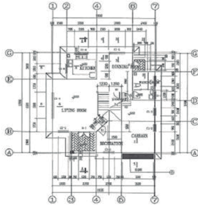
Plano
