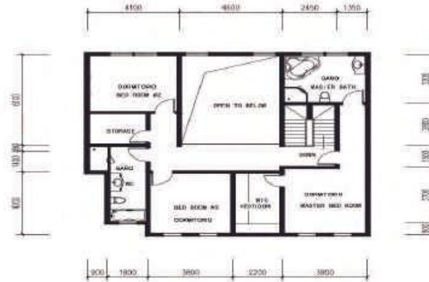
Plano Segunda Planta
