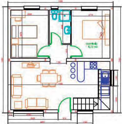
Plano Planta Baja
