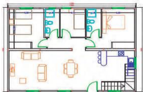
Plano Planta Baja
