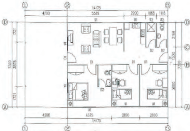
Plano
