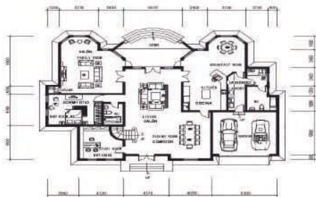
Primera Planta
