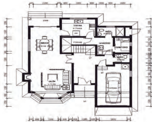
Plano Primera Planta
