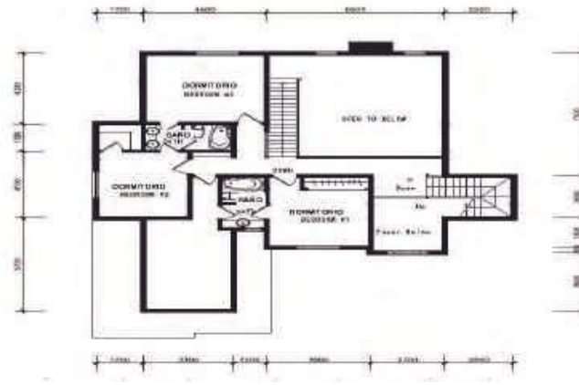
Plano Segunda Planta
