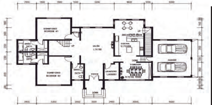
Plano Primera Planta
