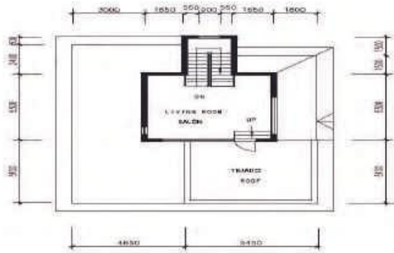
Tercer Planta
