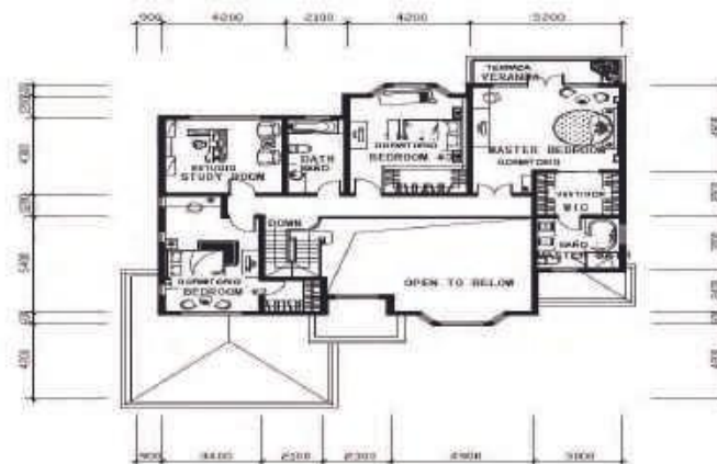
Plano Segunda Planta
