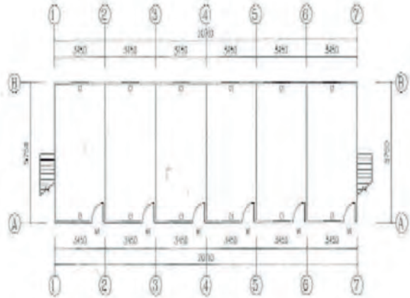
Primera Planta
