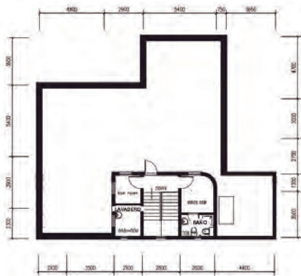
Tercer Planta
