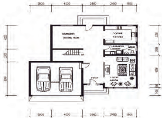
Plano Primera Planta
