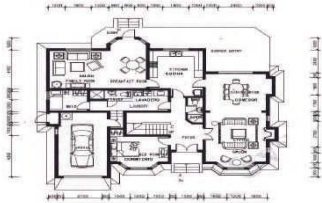
Plano Primera Planta
