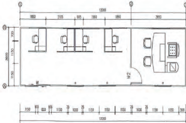
Plano
