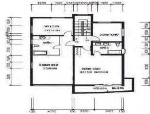
Segunda Planta
