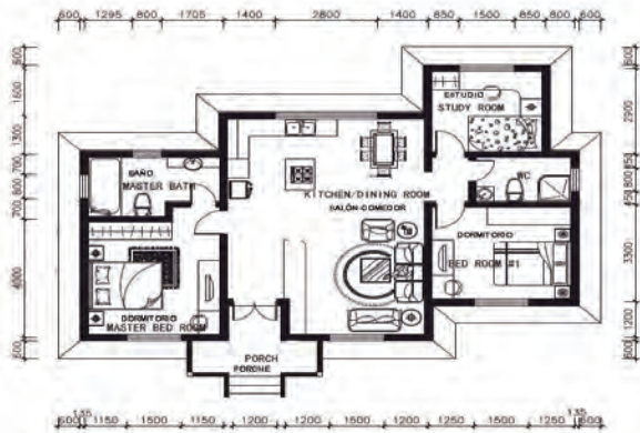
Plano
