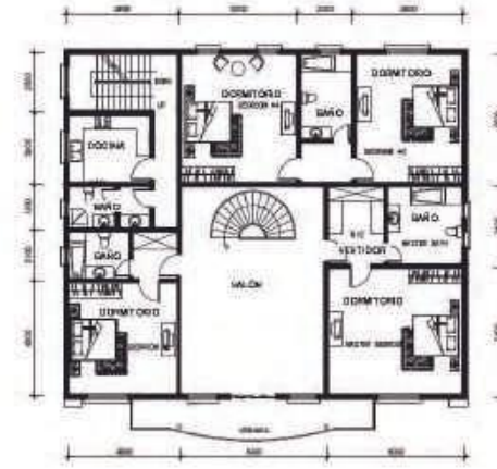
Segunda Planta
