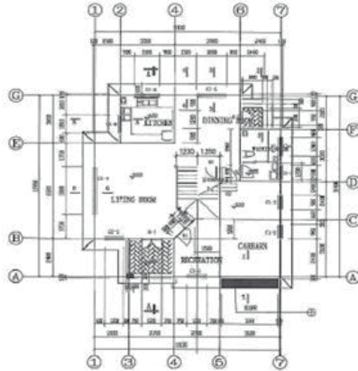
Plano
