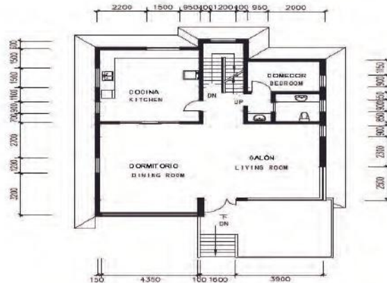
Primera Planta
