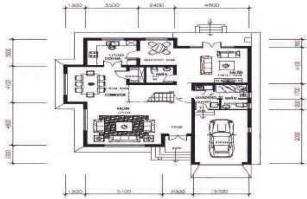
Plano Primera Planta
