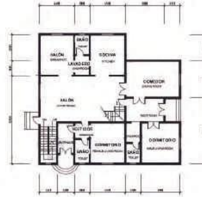
Primera Planta
