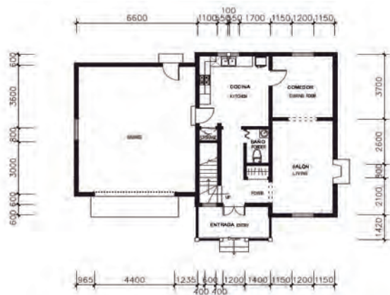
Plano Primera Planta
