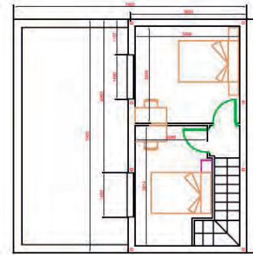
Plano Planta Alta
