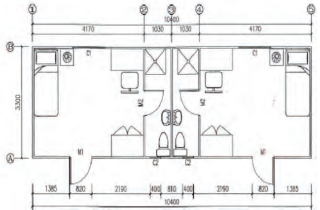
Plano
