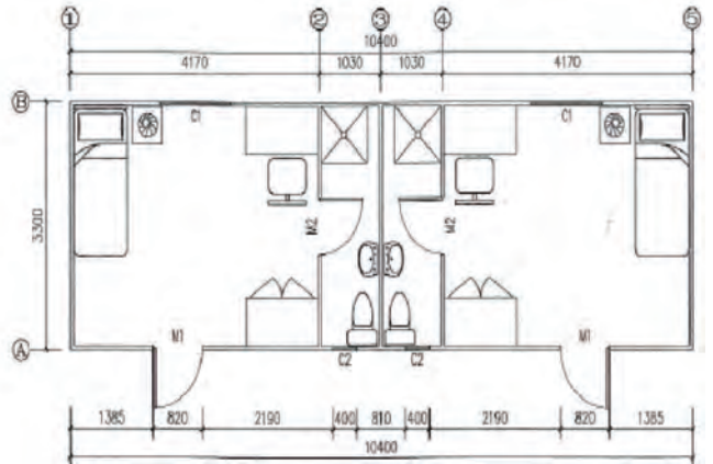
Plano
