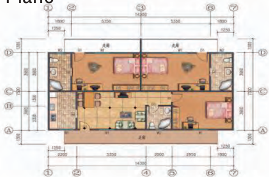
Plano
