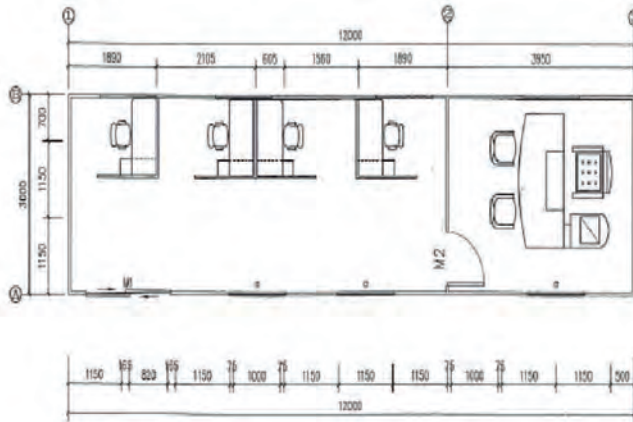
Plano
