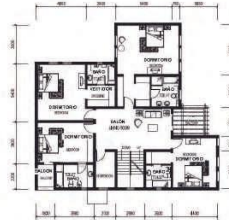
Segunda Planta
