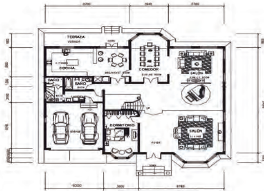
Plano Primera Planta
