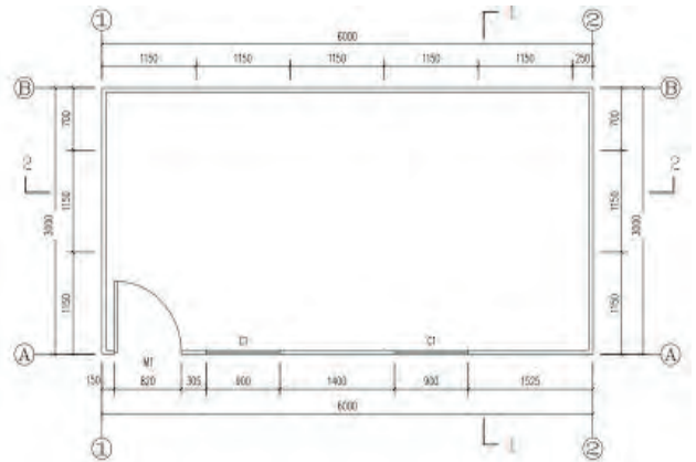
Plano
