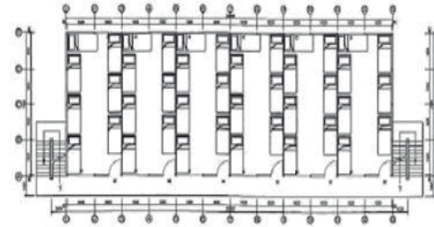
Segunda Planta
