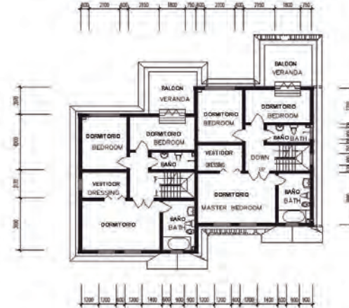
Segunda Planta
