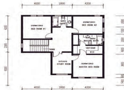
Plano Segunda Planta
