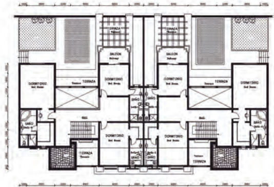
Segunda Planta
