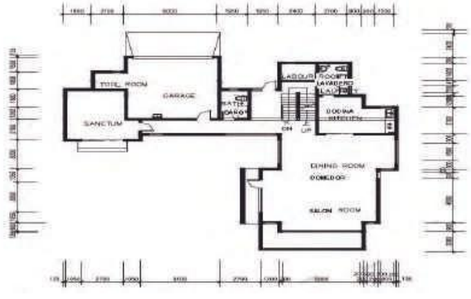
Plano Primera Planta
