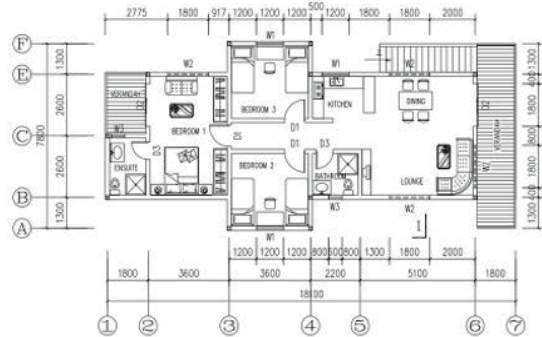
Plano
