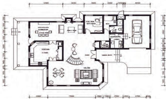
Plano Primera Planta
