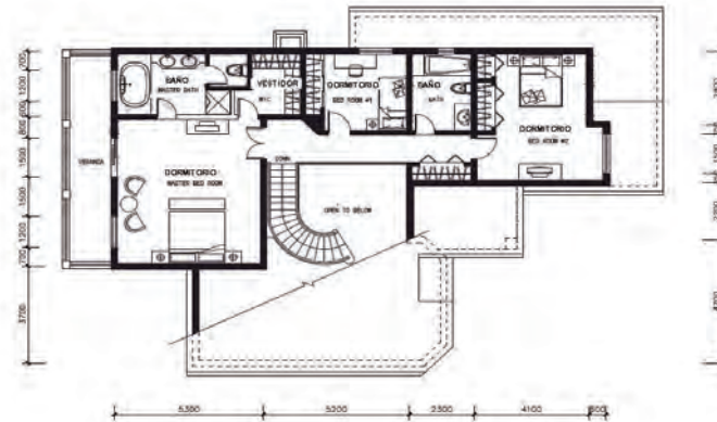
Plano Segunda Planta
