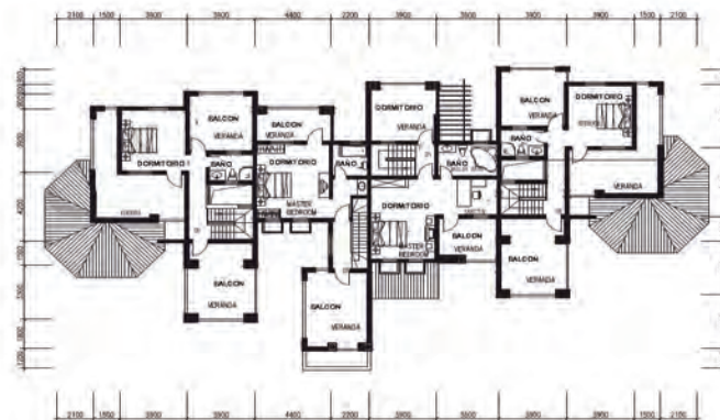
Tercer Planta
